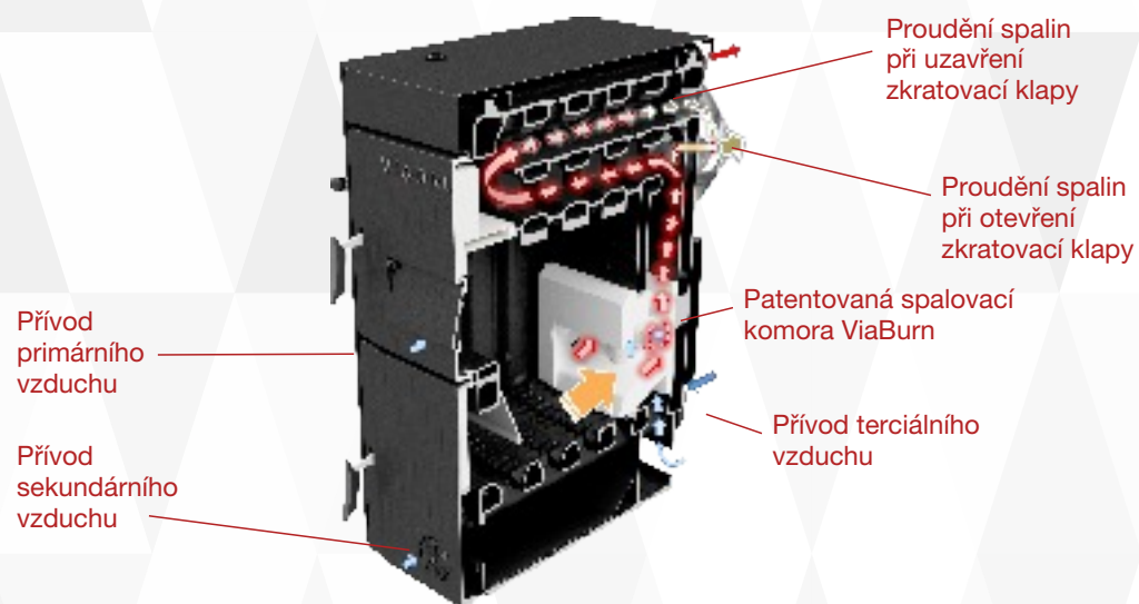
VIADRUS U22 Economy – Řez kotle - Schéma přívodu vzduchu a odvodu spalin
